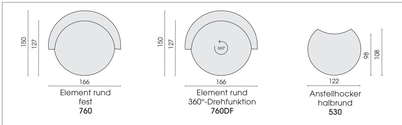
Seitenansicht
