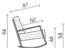
Seitenansicht
